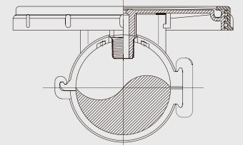
鞍座式安装
