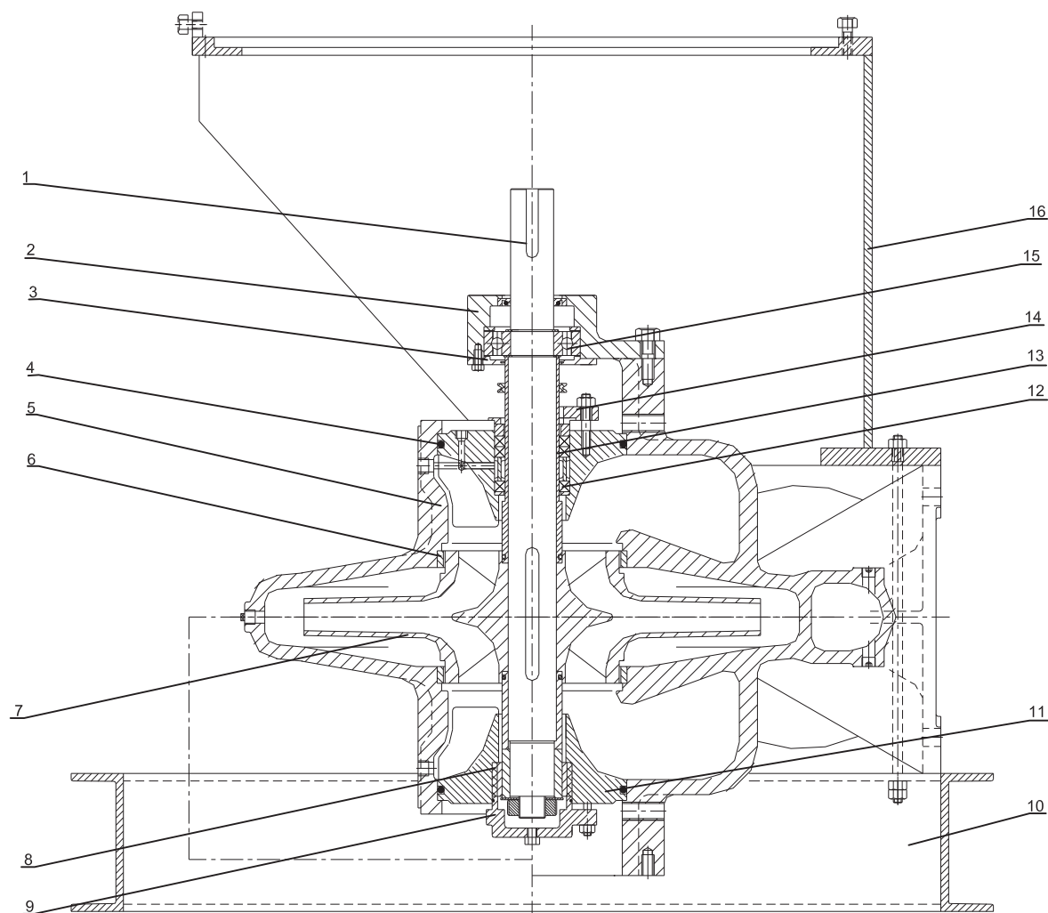
DV型立式泵结构图(DV80~DV350)
